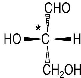
L-glycéraldéhyde
