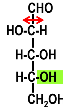
D-arabinose
