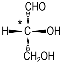
D-glycéraldéhyde
