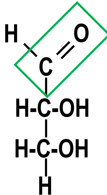
glycéraldéhyde (aldose)
