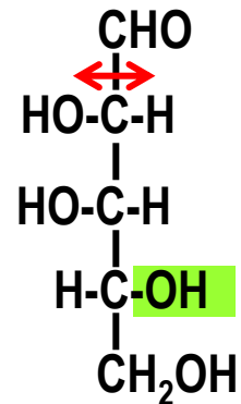
D-lyxose
