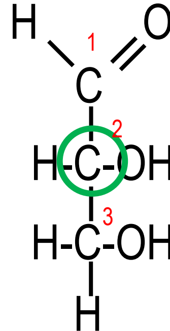
glycéraldéhyde (aldose)
