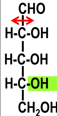
D-ribose
