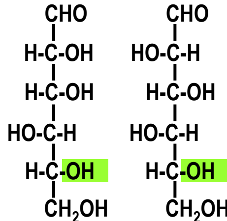
D-gulose
