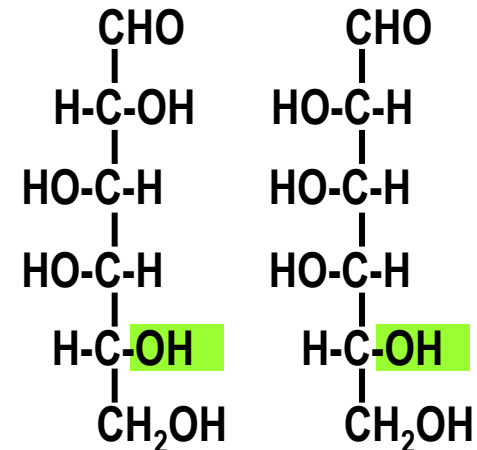
D-galactose
