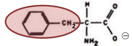
Phénylalanine (Phe)
