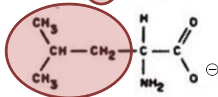
Leucine (Leu)
