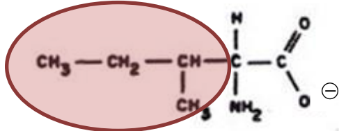
Isoleucine (Ile)
