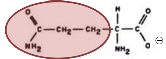
Glutamine (Gln)
